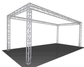
Carreconstructie 9 x 6 x 3,5 m
